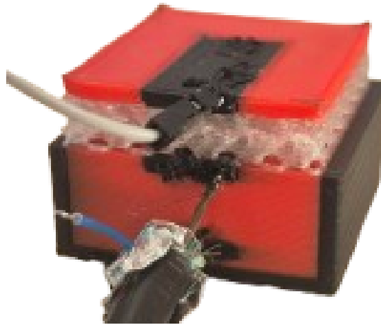
Figure 7. Design du capteur prenant en compte la réduction des plaques pour limiter l'impact du shield sur la mesure.
