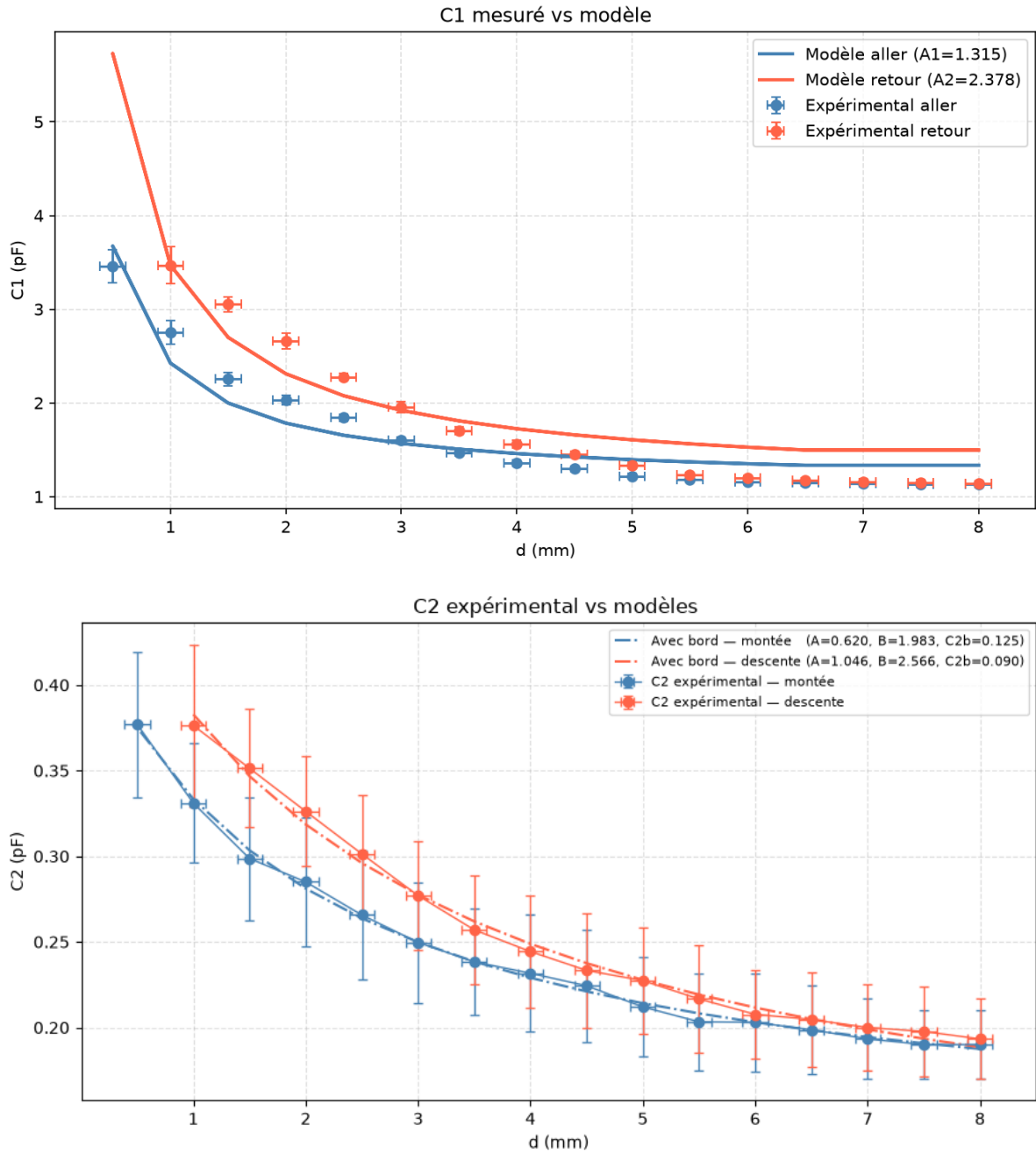
Figure 9. On peut voir que le modèle de C_1 n'est pas très précis, mais pour un capteur que l'on veut peu coûteux, on peut accepter une grande incertitude. De plus, si l'on a les valeurs des constantes, une seule mesure suffit ; et comme celle de C_2 paraît meilleure, on pourrait exploiter celle de C_2 .
